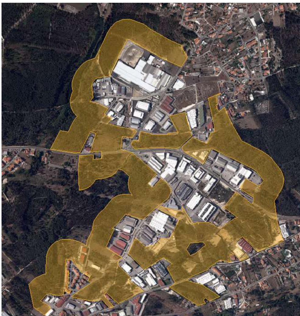
Fig. 12 - Faixa de gestão de combustível junto da Zona Industrial da Marinha Pequena (ZIMP)
